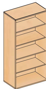
KNR80-308 →80 ↑186 ↗42
