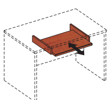
KNX10-308 →67,5↑8↗40
