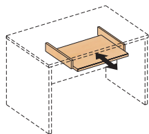
KNX10-308 →67,5 ↑8 ↗40
