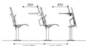
chair setting mode Aufstellung der Bestuhlung
